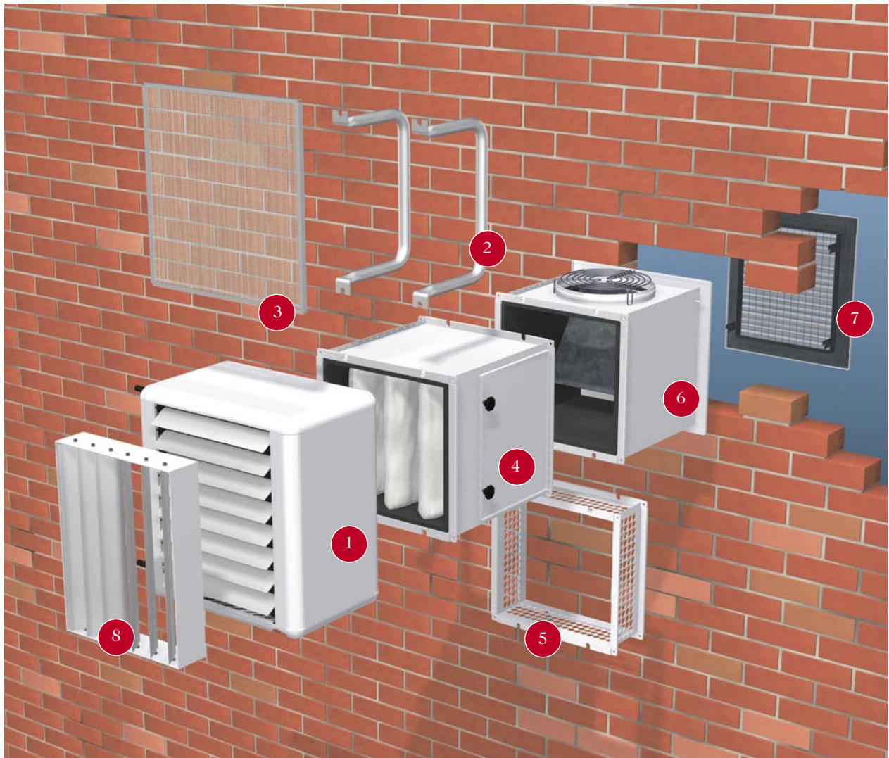
1) Тепловентилятор SW 2) Монтажные скобы SWK 3) Сетчатый воздушный фильтр SWFT 4) Секция фильтра тонкой очистки воздуха SWF 5) Секция рециркуляции SWD 6) Камера смешения SWBS 7) Решетка для отверстия в стене SWY 8) Дополнительные жалюзи SWLR.
