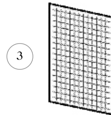
1) Тепловентилятор SW 2) Монтажные скобы SWK 3) Сетчатый воздушный фильтр SWFT 4) Секция фильтра тонкой очистки воздуха SWF 5) Секция рециркуляции SWD 6) Камера смешения SWBS 7) Решетка для отверстия в стене SWY 8) Дополнительные жалюзи SWLR.
