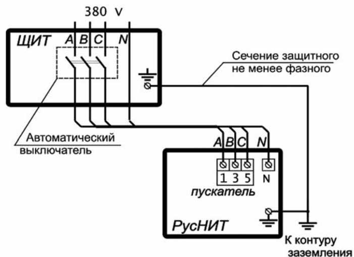
Рис.8. Схема подключения РучНИТ-206М, 207М, 208М, 209М к трехфазной сети.
