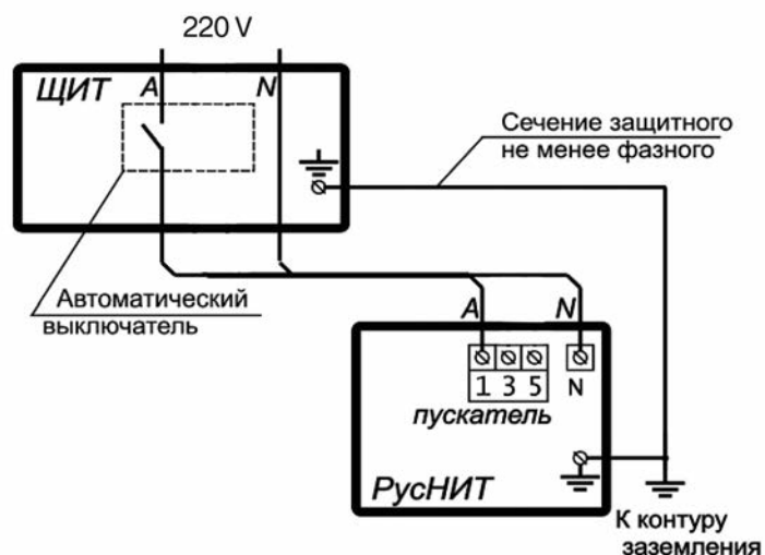
Рис.7. Схема подключения к однофазной сети РучНИТ-205М (206М, 207М, 208М, 209М - с использованием пластины РУСН.741124.067).
