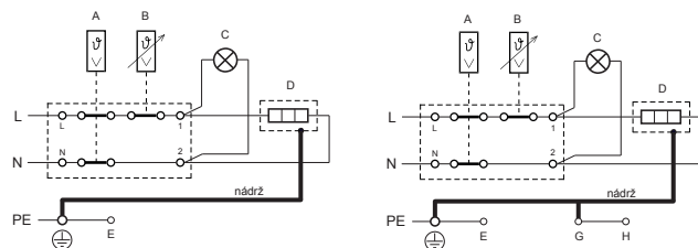
Рис. 5: Схема электрического подключения
